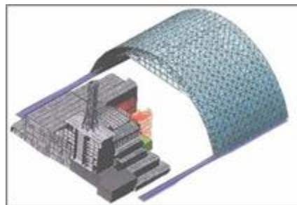
Конструкція конфайнменту Чорнобильської АЕС
